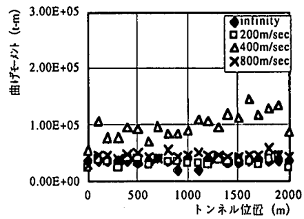
図-15 鉛直方向加震時の曲げモーメント分布 (Type-C)
