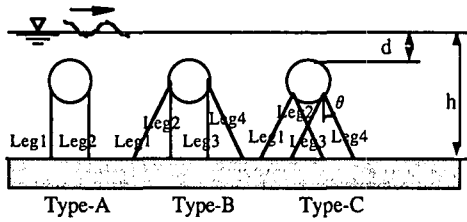
図-2 係留索配置
