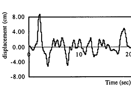
図-10 地震変位波形（水平方向）
