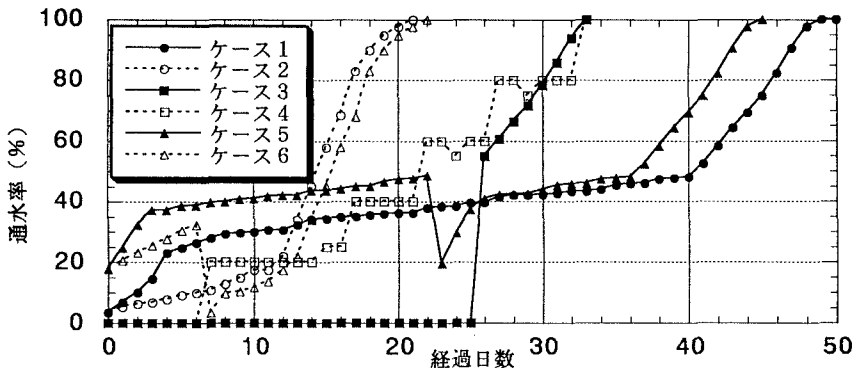
図-3 通水率の変化
