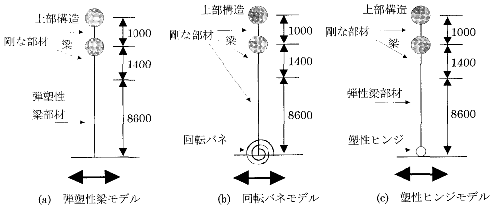
図2 解析モデル
