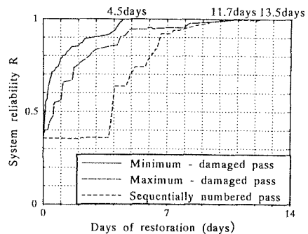
図6 戦略の違いによる復旧日数のシミュレーション
