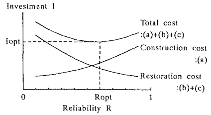
図1 投資と信頼性の関係
