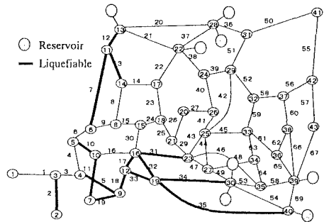
図2 熊本市上水道幹線網のモデル化
