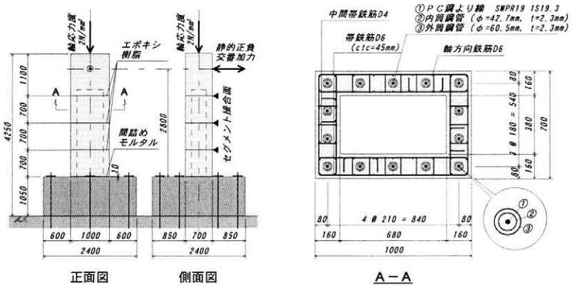
※1 柱部分とフーチング部分は同じコンクリートを使用している。 ※2 内筒鋼管は柱頭部からフーチング下面まで貫通して配置してある。 ※3 外筒鋼管はセグメント接合面で分断されている。
