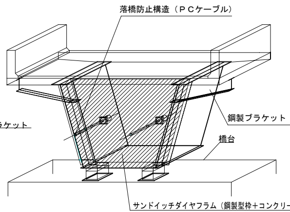
図-2 サンドイッチダイヤフラム
