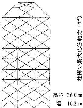
図6 解析モデルC
