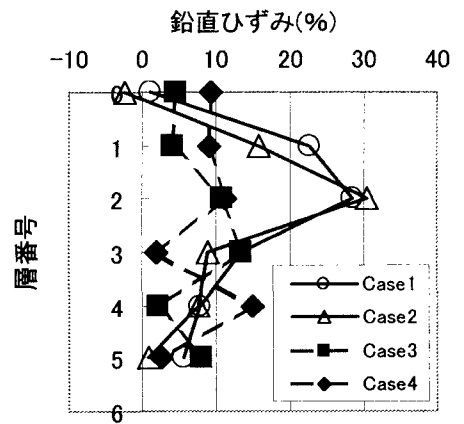
図 4 層別鉛直ひずみ
