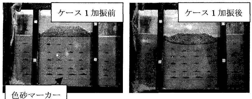
図 2 実験模型および変形状況
